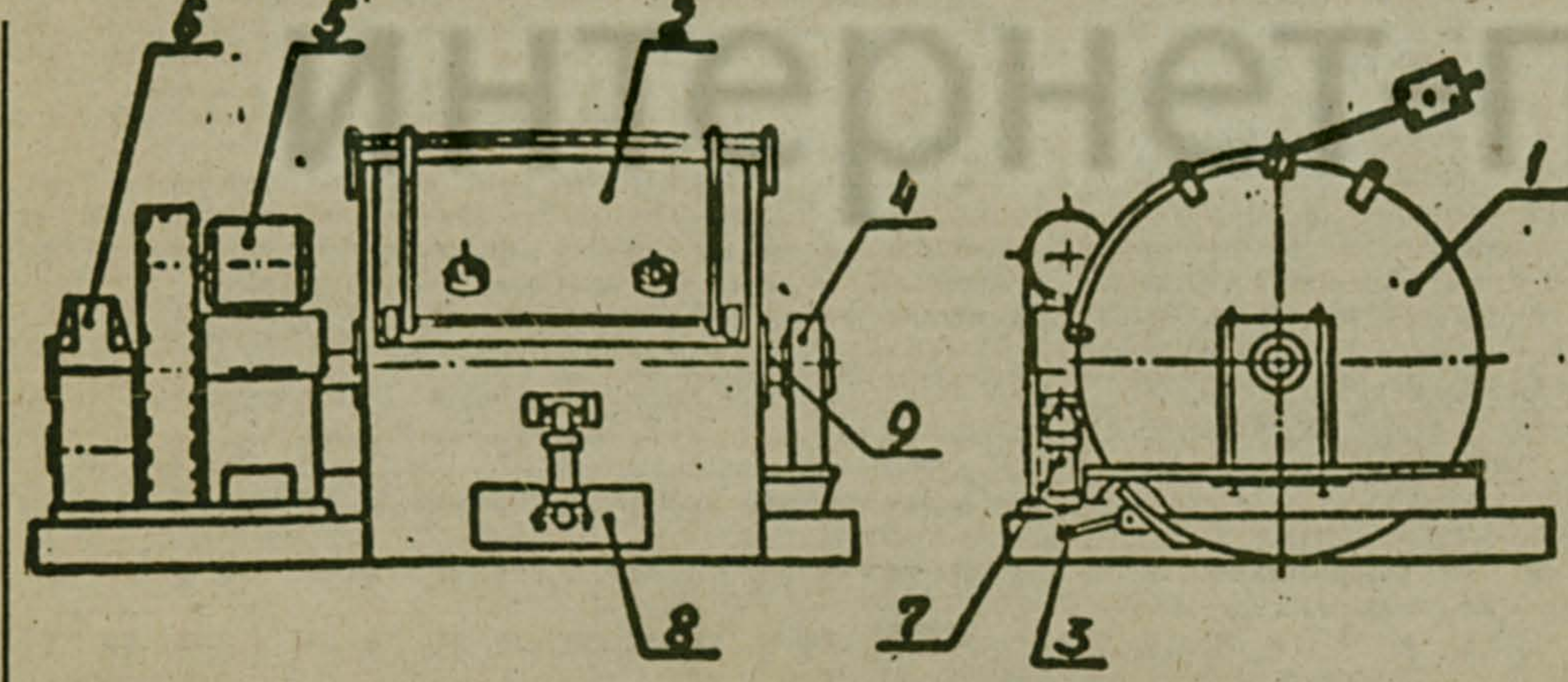
На рис. бетономеситель: 1 — корпус; 2 — крышка; 3 — затвор; 4 — опора; 5 — электродвигатель; 6 — редуктор; 7 — пневмоцилиндр; 8 — люк для выгрузки; 9 — вал рабочий.
