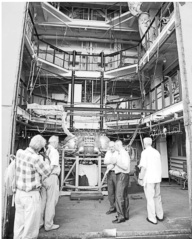
НИЦ РКП имеет уникальную стендовую базу, позволяющую проводить испытания любой космической техники, в том числе тяжелых ступеней ракет с двигателями большой тяги. Этот подмосковный «космодром» дает путевку в жизнь новым космическим разработкам.
