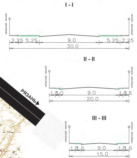
ПОПЕРЕЧНЫЕ ПРОФИЛИ УЛИЦ (М 1: 200)
